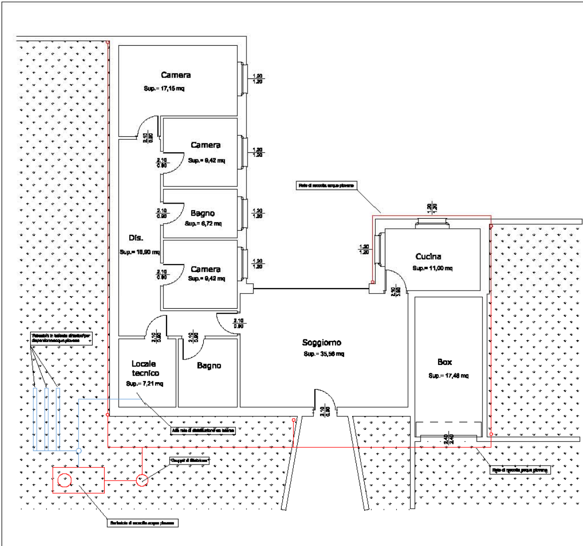
SCHEMA RETE DI RACCOLTA ACQUE METEORICHE
